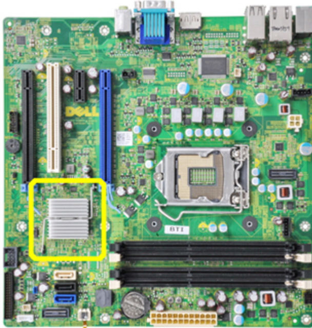
Abbildung 1. Systemplatine einer früheren Version mit dem Kühlkörper
