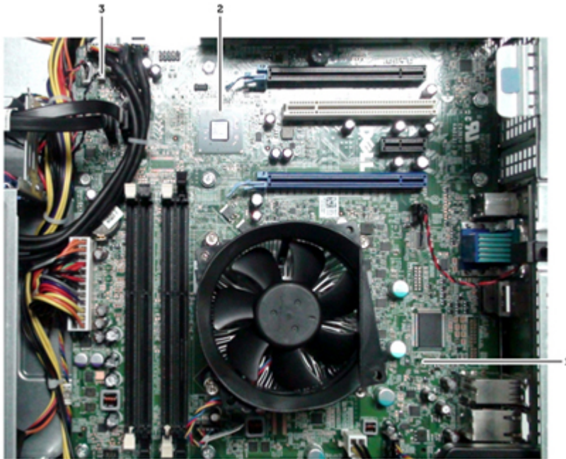
Abbildung 2. Systemplatine mit entferntem Thermosensor und Kühlkörper
